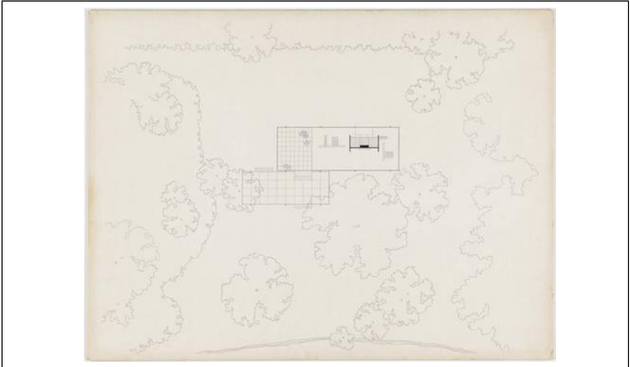
Figura 05 – Planta da Casa Farnsworth
